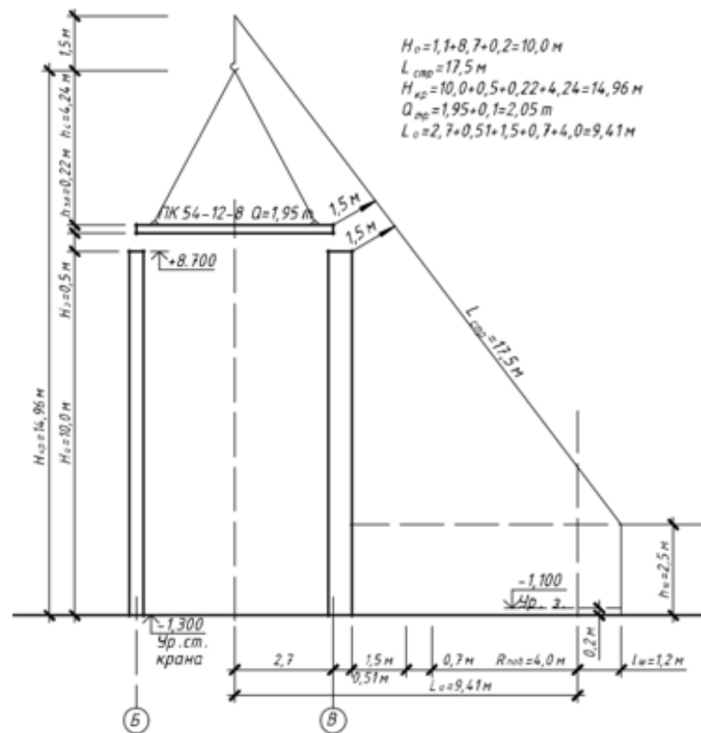
Рисунок 1.6 – Схема определения рабочих параметров крана
