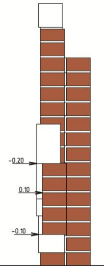
Разрез 1-1 М 1:15
