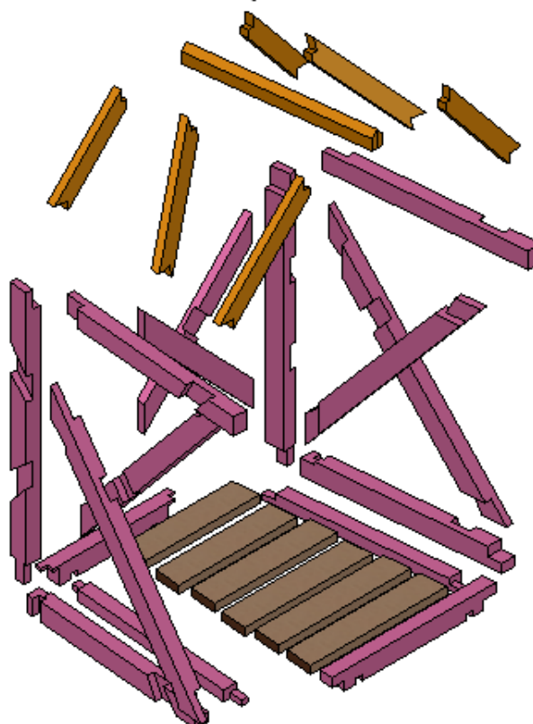
Взрыв-схема
